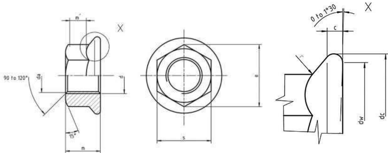
Dimensions of Metric DIN 6923 Hexagon Flange
